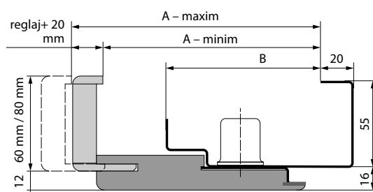
SECȚIUNE TOC PROIECT PREMIUM
