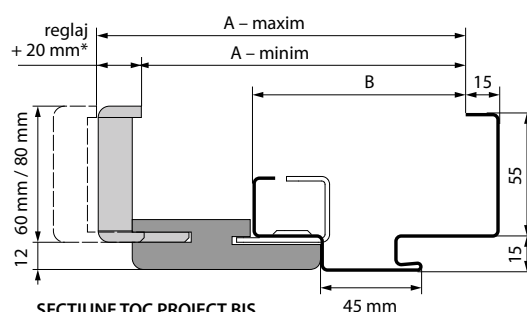
SECȚIUNE TOC PROIECT BIS
